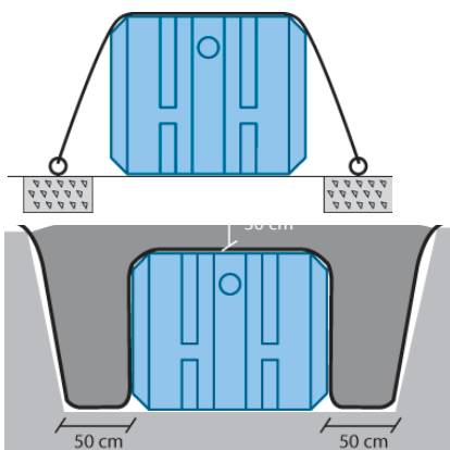
Eksempel på forankring i betong eller fjellgrunn.
